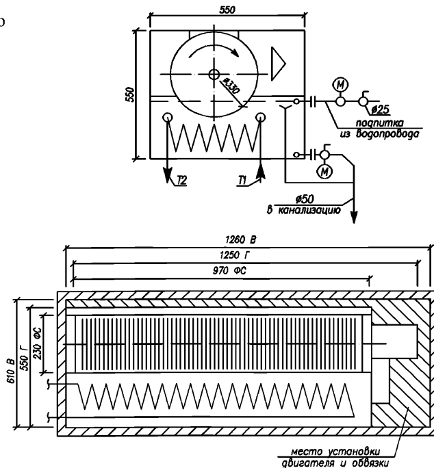
Рисунок 10.14 – Компонировочный чертеж РПУТ330з
