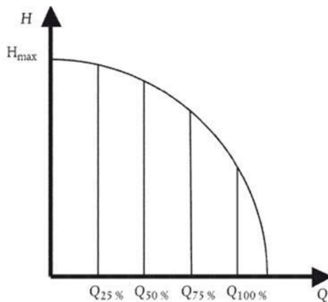
Рис. 3. Профиль нагрузки.
