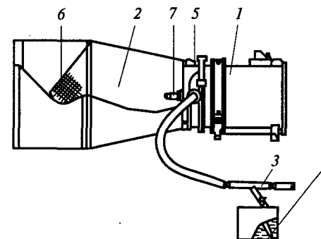
Рис. 8.5. Пеногенераторная установка ПГУ-200:
