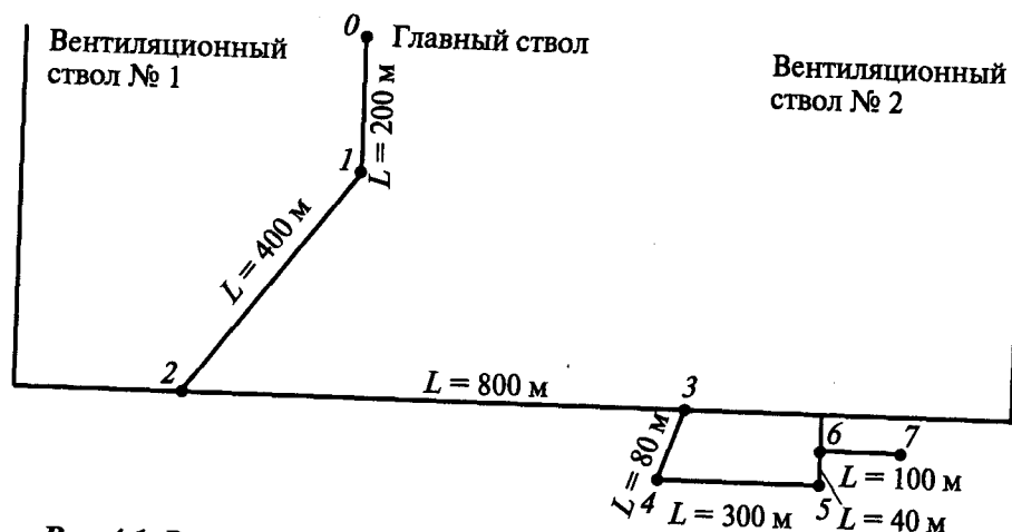
Рис. 4.1. Расчетная схема ветви пожарно-оросительного водопровода
