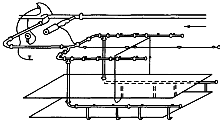
Рис. 8.13. Установка автоматического пожаротушения УАП
