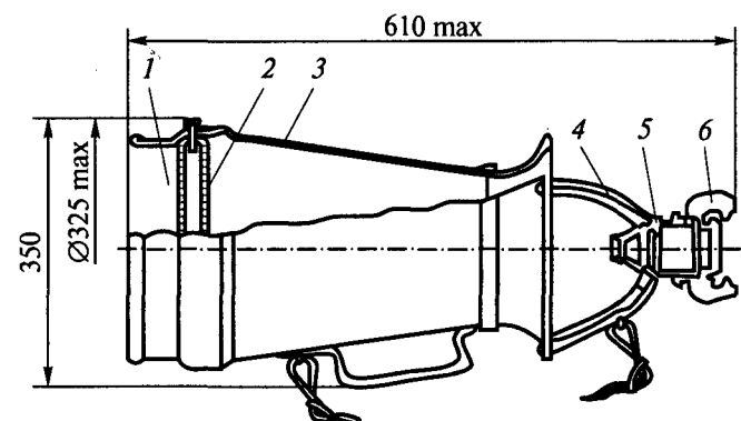
Рис. 8.6. Генератор пены средней кратности ГПС-600:
