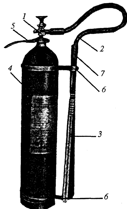
Рис. 8.1. Огнетушитель ОУ-8: 1 — вентиль; 2 — шланг; 3 — диффузор; 4 — баллон; 5 — рукоятка; 6 — скобы для крепления диффузора; 7 — ручка диффузора
