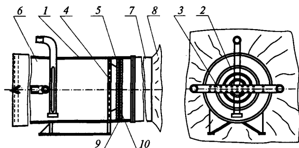
Рис. 8.3. Пеногенератор НПУ-0,5:
