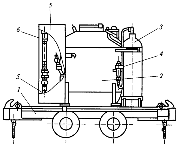
Рис. 8.9. Установка УП-250:
