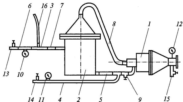
Рис. 8.4. Установка высоконапорная пеногенераторная ВПГУ-0,2:
