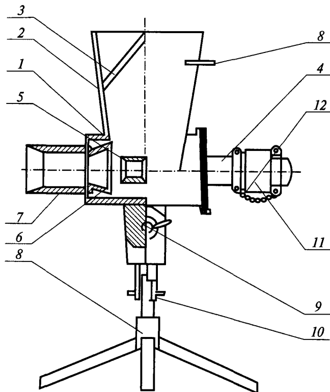
Рис. 8.8. Установка порошковая шахтная эжекционная УПШЭ: 1 — корпус; 2 — приемный бункер; 3 — нож; 4 — труба для подачи воздуха; 5 — сопло; 6 — конфузор; 7 — распылитель; 8 — подставка; 9 — механизм поворота; 10 — стопор; 11 — подсоединительная муфта; 12 — предохранительная цепь
