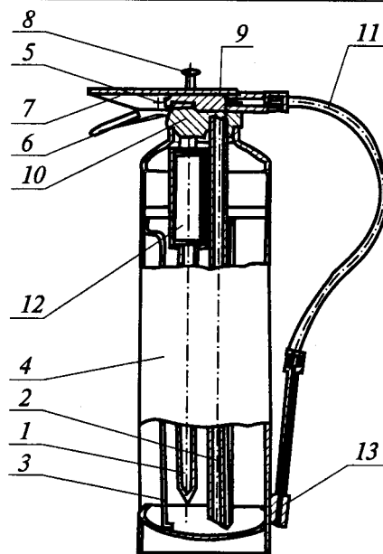
Рис. 8.2. Огнетушитель типа ОП-Г:
