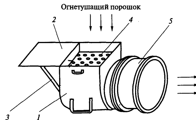
Рис. 8.7. Установка порошкового пожаротушения УПП-3: 1 — корпус; 2 — крышка-стол; 3 — стойки; 4 — дозирочная решетка; 5 — вентилятор
