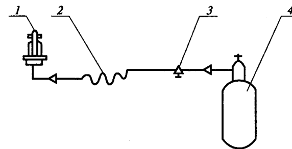
Рис. 8.11. Схема испытания предохранительного клапана:
