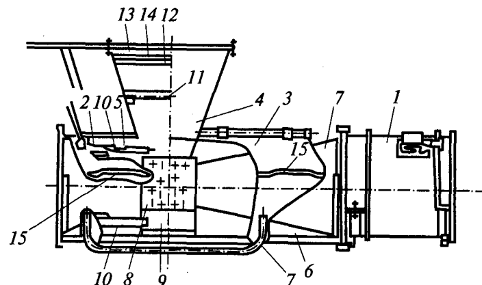
Рис. 8.12. Устройство «Вихрь»:
