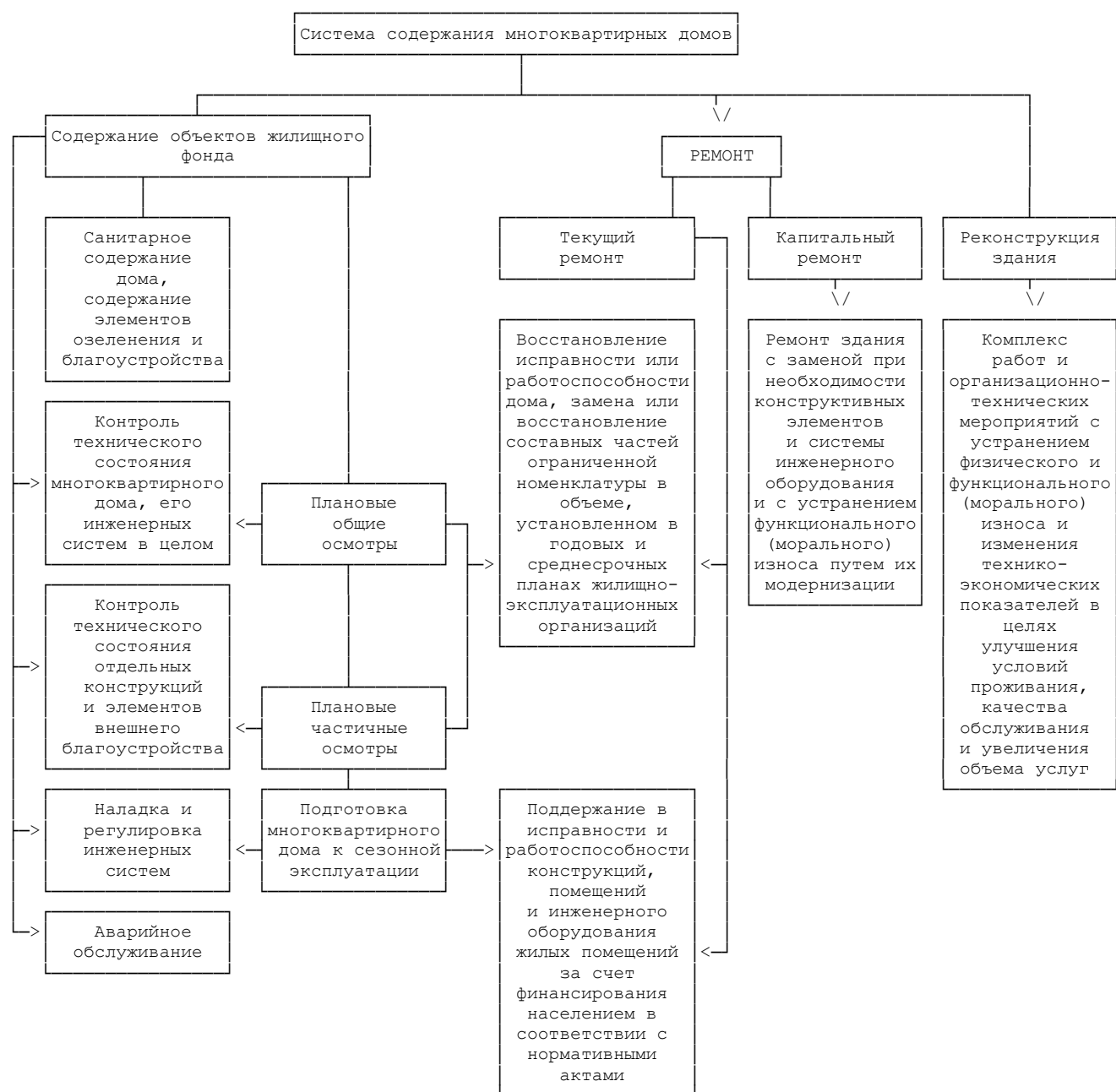
Рис. 1.1. Принципиальная схема системы содержания многоквартирных домов с учетом "Правил содержания общего имущества в многоквартирном доме", утвержденных Постановлением Правительства Российской Федерации от 13 августа 2006 года N 491
