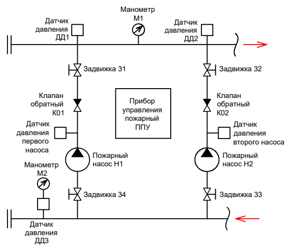
Общая принципиальная схема установки Hydro MX-V
